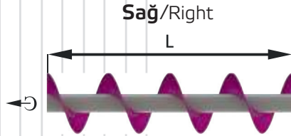
St37 Çekme Helezon Standart Ölçüleri Dimension Table St37
