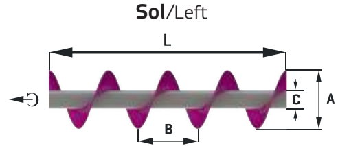
304-316 Çekme Helezon Standart Ölçüleri Dimension Table AISI316
